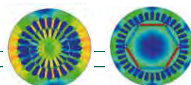
Motor Inducción
