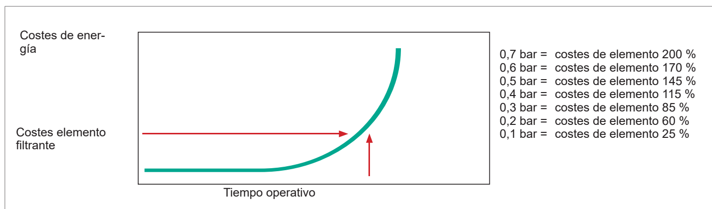
Fig.: Trascuro típico de presión diferencial, costes de energía en relación con los costes del elemento filtrante
